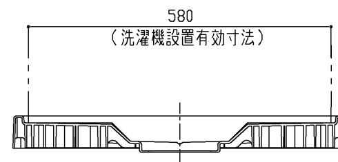
断面B-B
