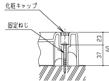
固定部詳細(尺度フリー)
