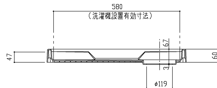
断面A-A
